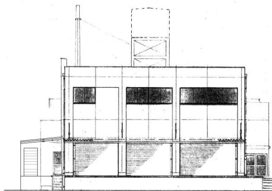
南立面图 1/100
