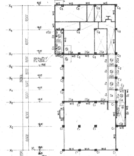
Z2 伏図 1/200
