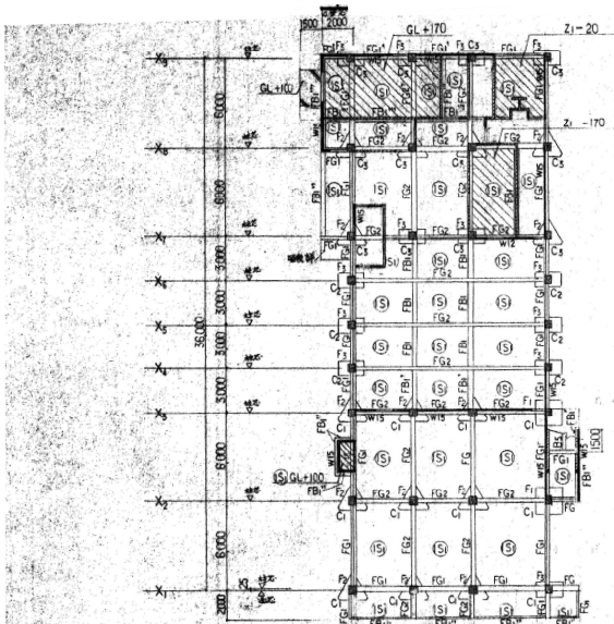
基盤伏図 1/200
