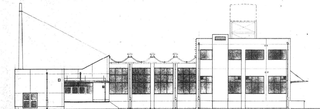
西立面图 1/100
