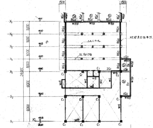
Z4 伏図 1/200
