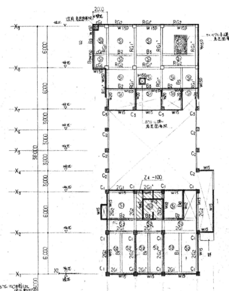
Z3, Z4 伏図 1/200
