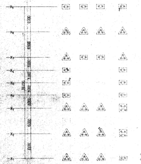
Z1 伏図 1/200
