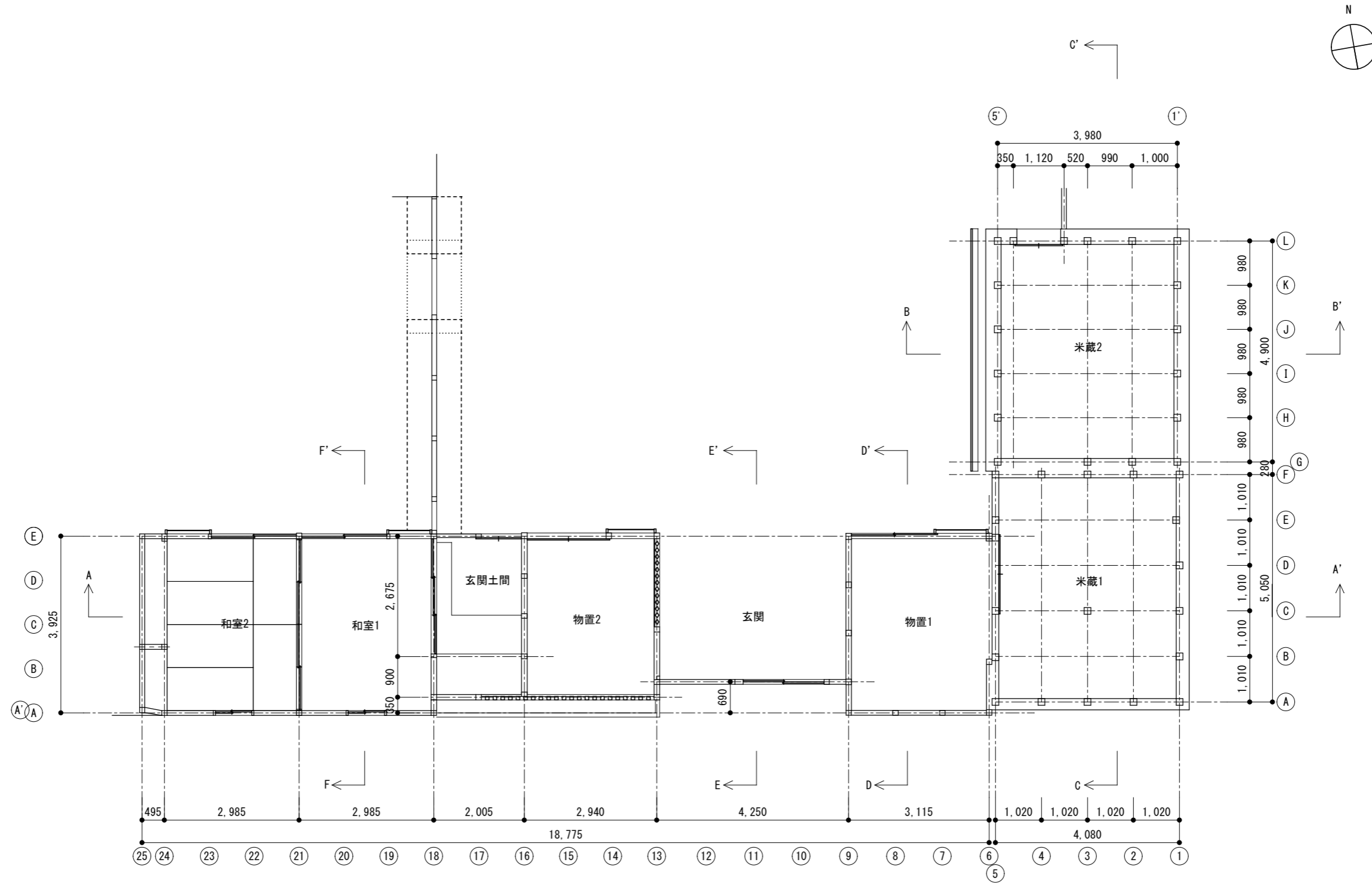
長屋門 現況平面図
