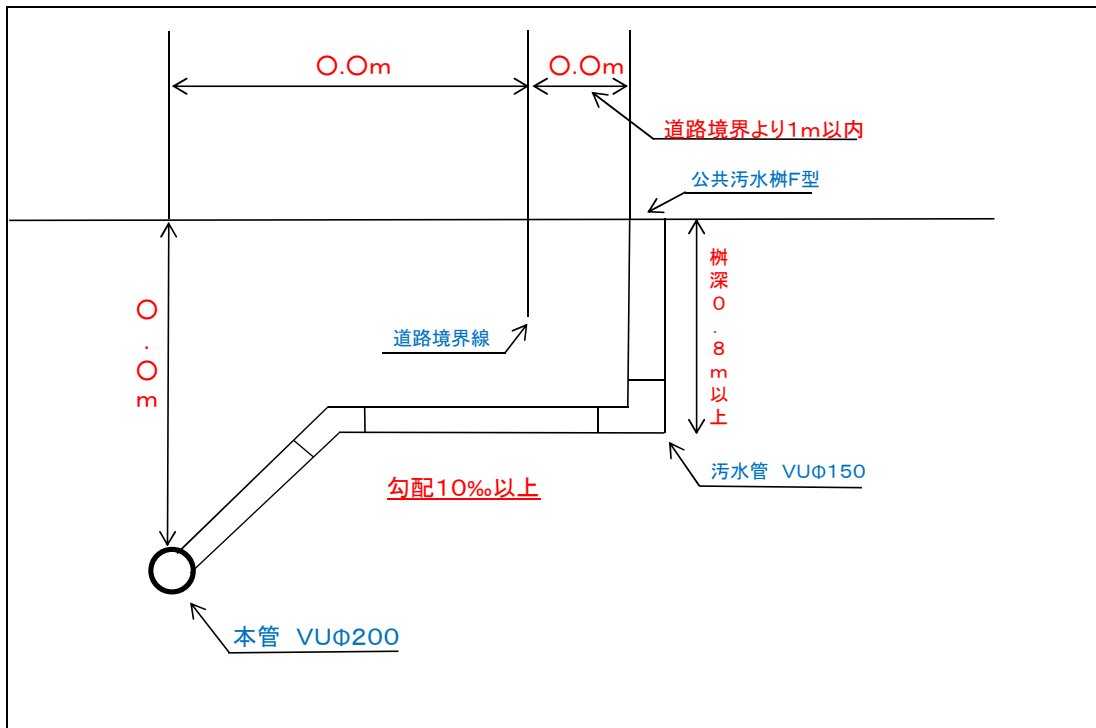
(断面図)
