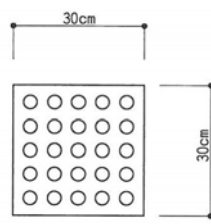
点状ブロック
