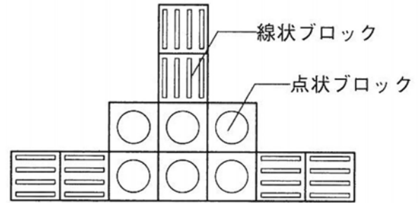
(例) 階段接続部の点状ブロック
