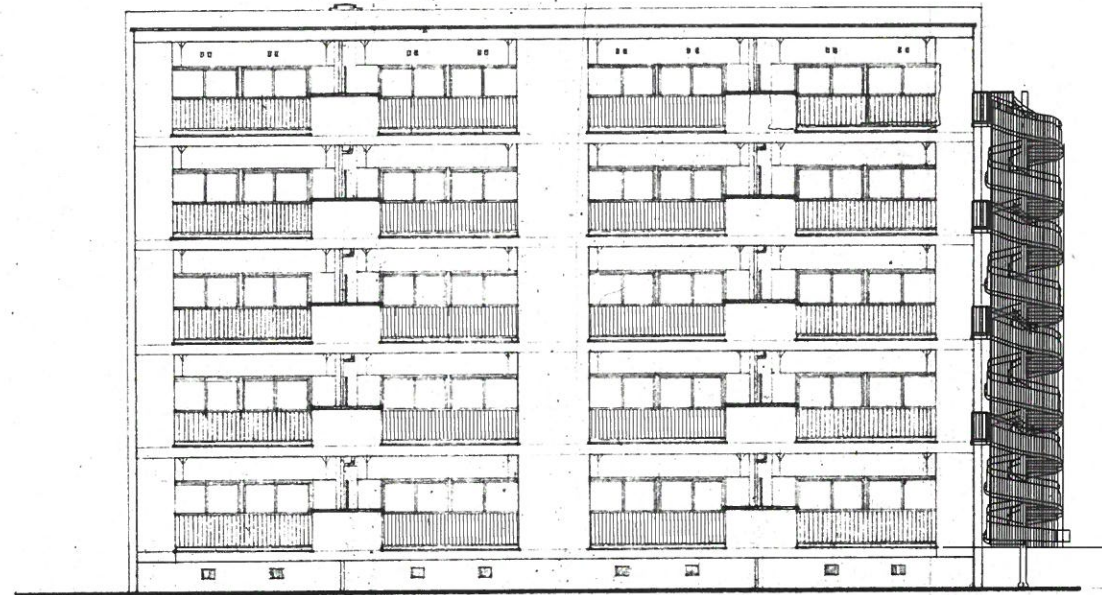
東立面図
