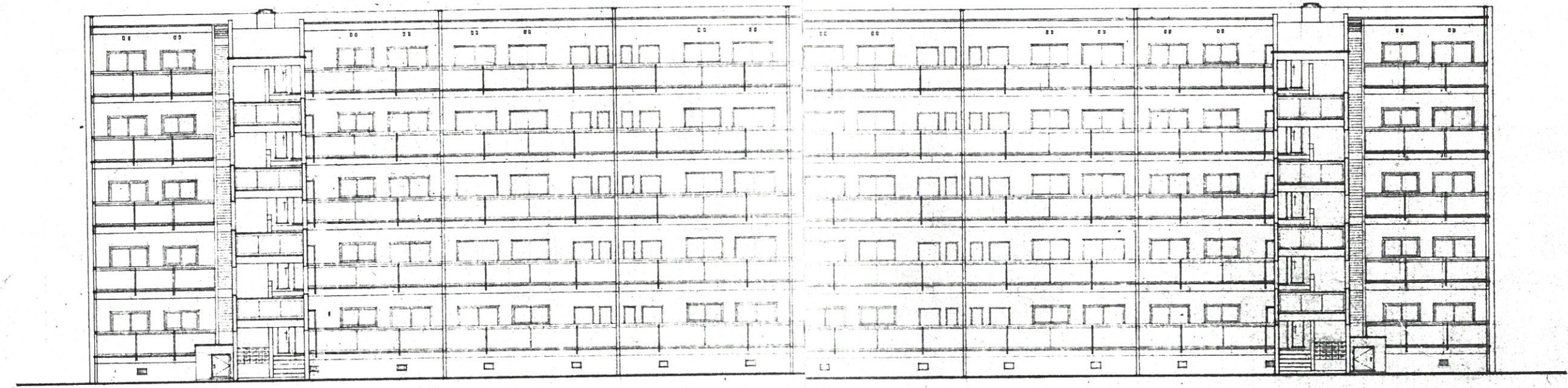
西立面図
