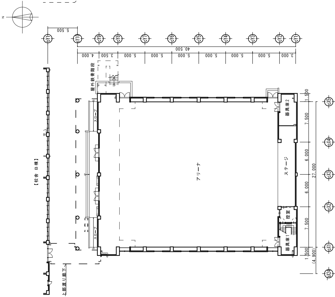
2階平面図
